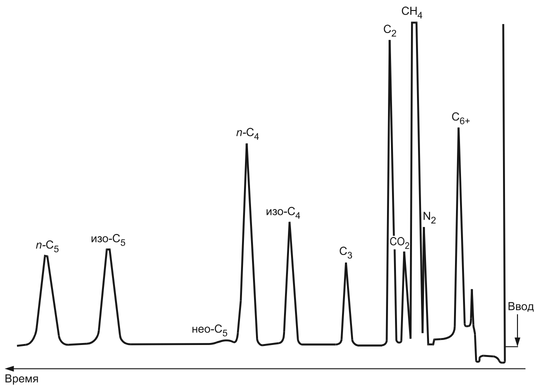
Рисунок 2 — Пример типичной хроматограммы
