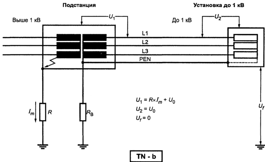
Рисунок 44В — TN-системы
